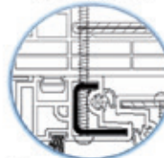
3 Stahlverstärkung im Mittelstoß
