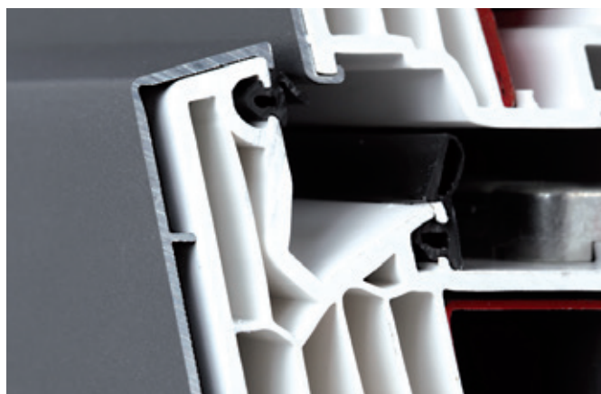
Die Wanddicke des Profils classica von 3 mm entspricht der höchsten Güteklasse Klasse-A.
