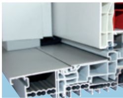
Thermisch getrennte Aluminium-Kunststoff-Schwelle.
